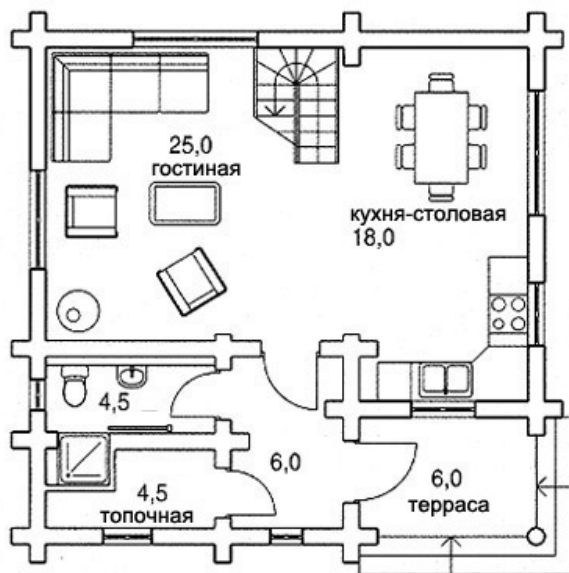
План 1 этажа
