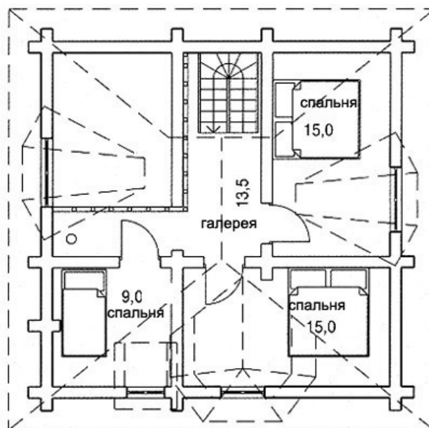
План 2 этажа
