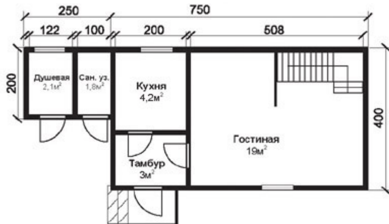
ПЛАН ПЕРВОГО ЭТАЖА
