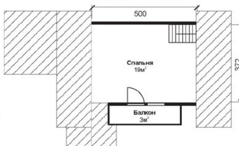
ПЛАН ВТОРОГО ЭТАЖА
