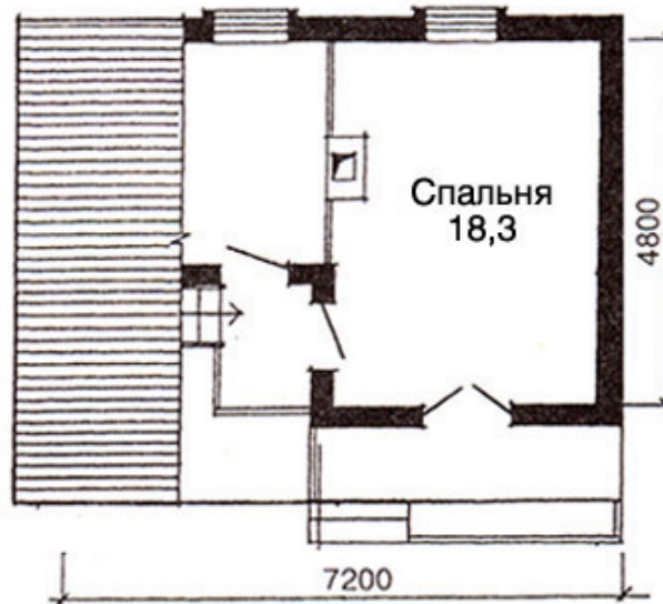
ПЛАН МАНСАРДЫ
