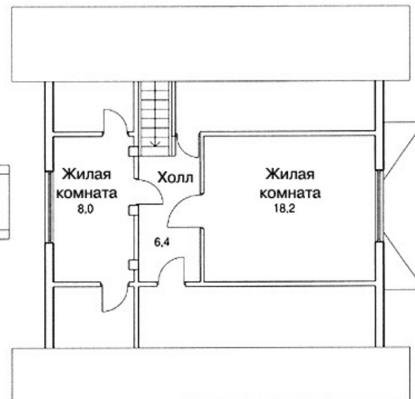
План 2 этажа
