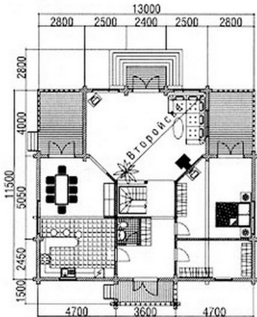
план 2 этажа
