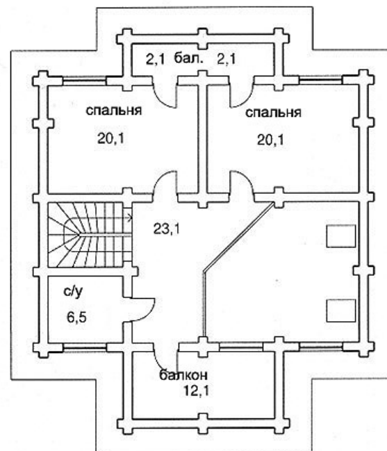
План 2 этажа
