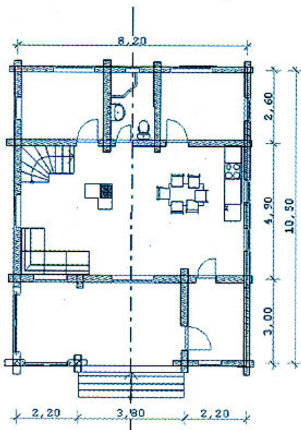
План 1 этажа
