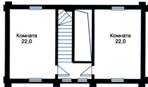
План 2 этажа
