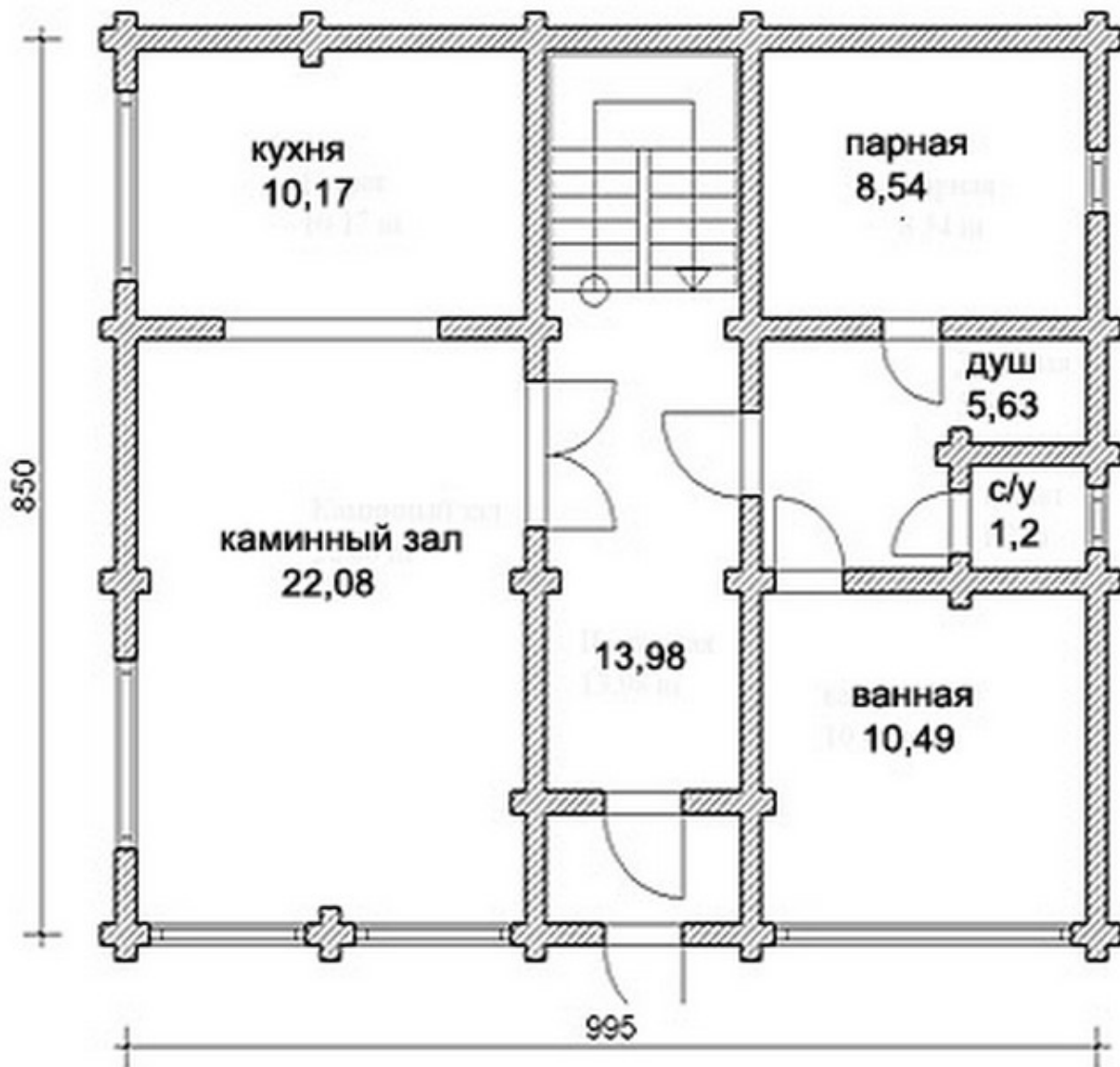
План 1 этажа
