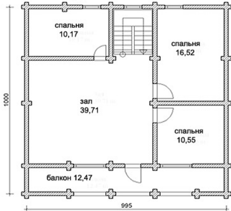
План мансарды
