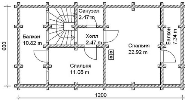
План мансарды
