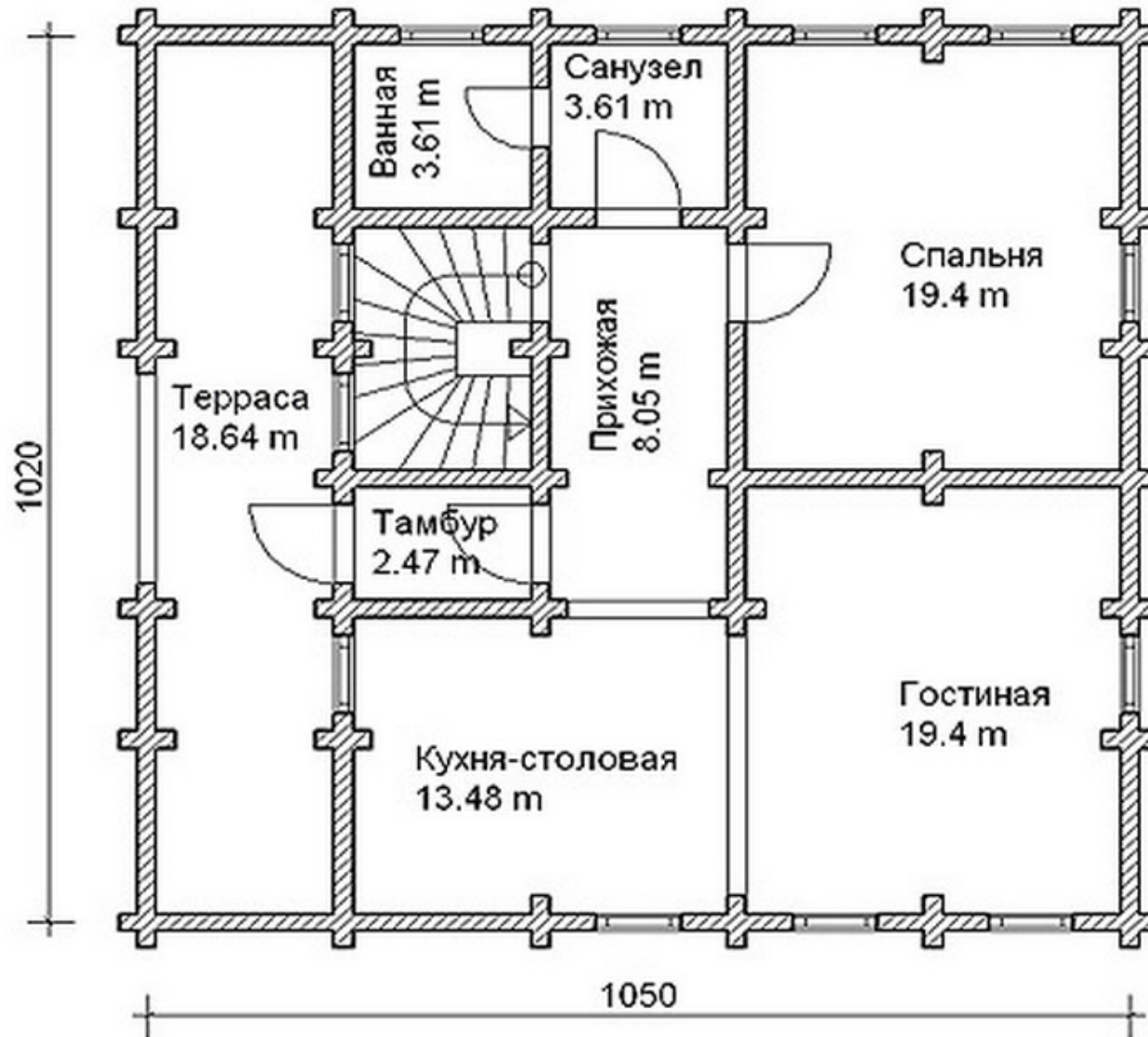
План 1 этажа
