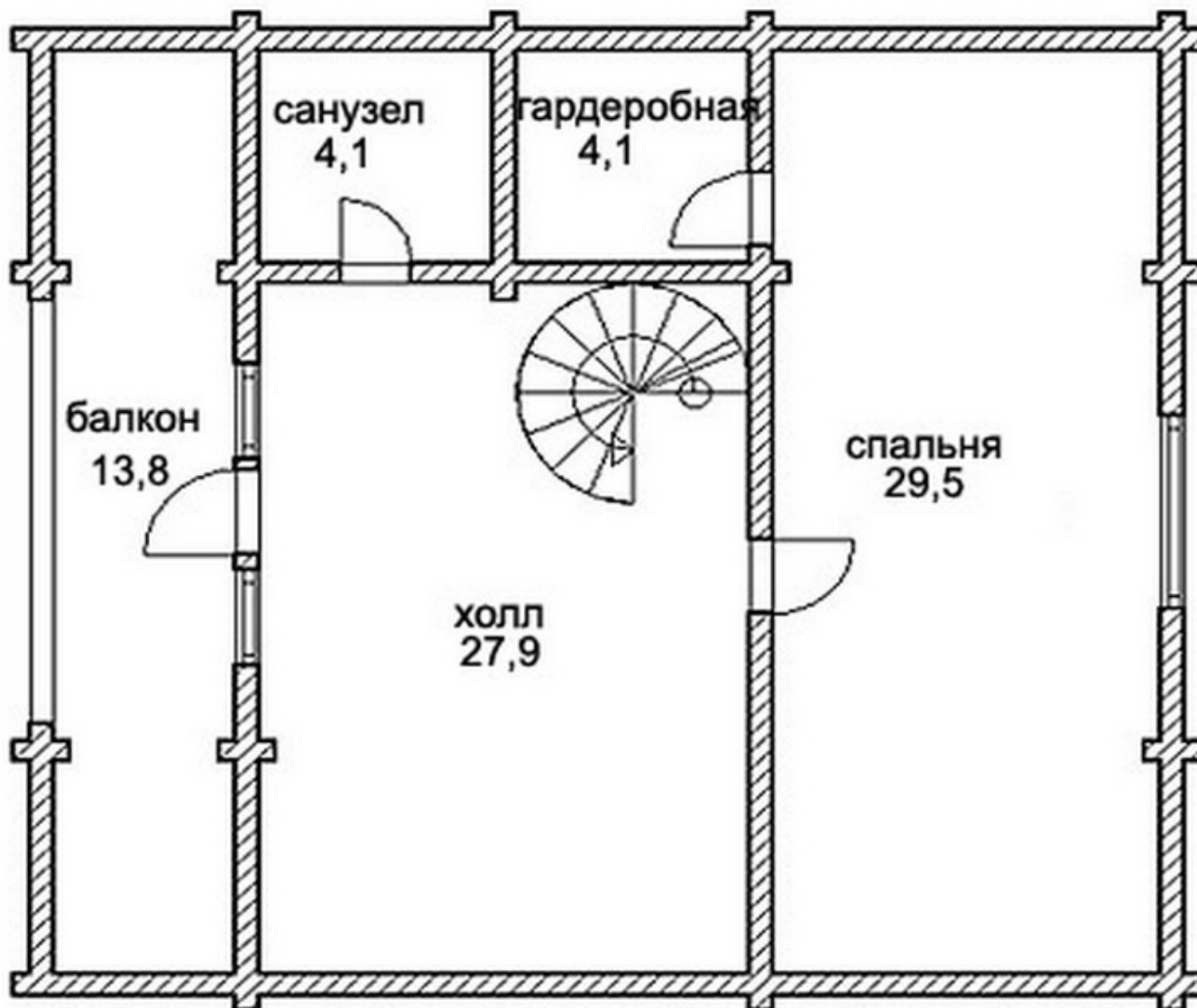
План 2 этажа
