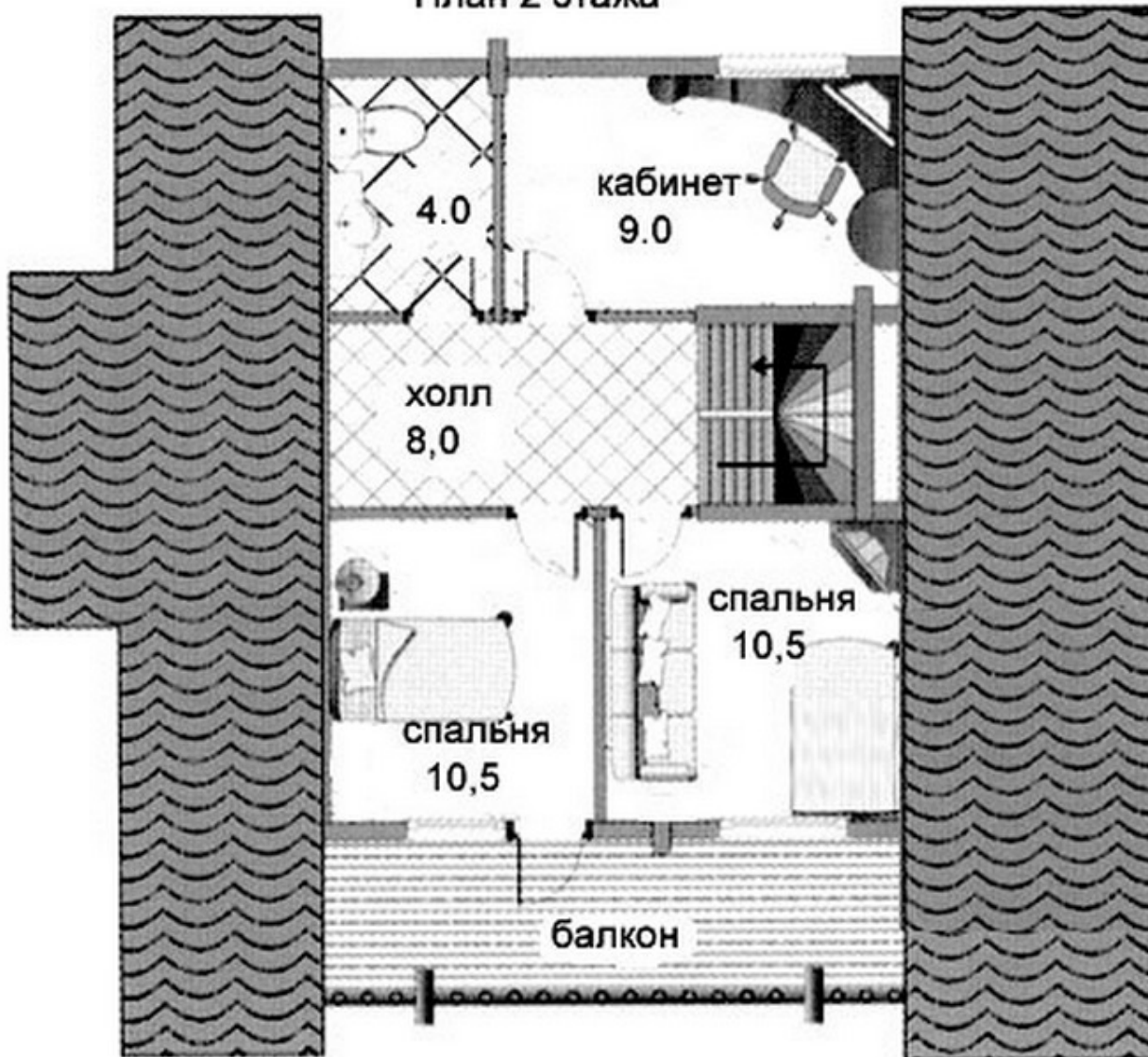
План 2 этажа
