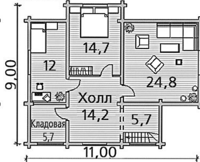
План 2 этажа
