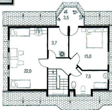
План 2 этажа
