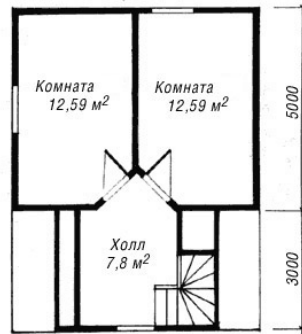
план второго этажа
