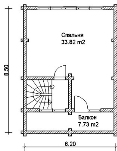
ПЛАН МАНСАРДЫ
