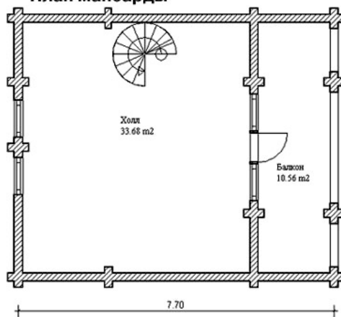
План мансарды
