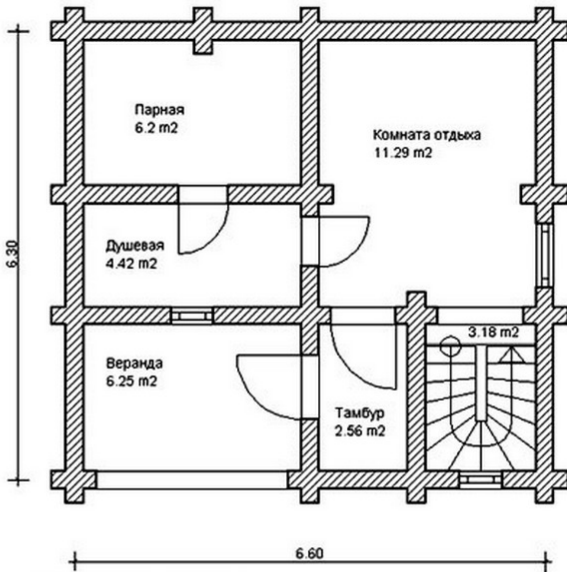
ПЛАН 1-ГО ЭТАЖА
